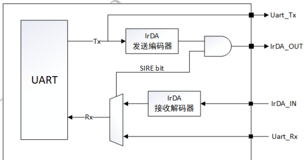
图 5-1 IrDA 框图
