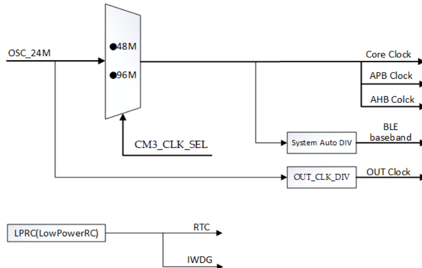
图 2-1 系统时钟树
