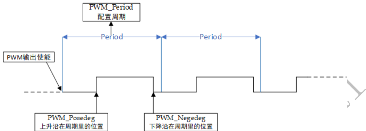
图 13-2 PWM 时序图
