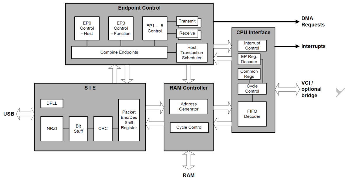
图 18-1 USB 系统框图
