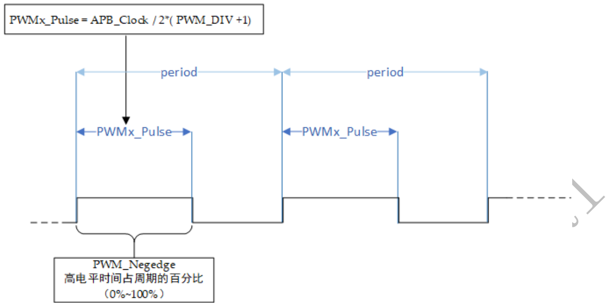
图 13-3 PWM_DAC 时序
