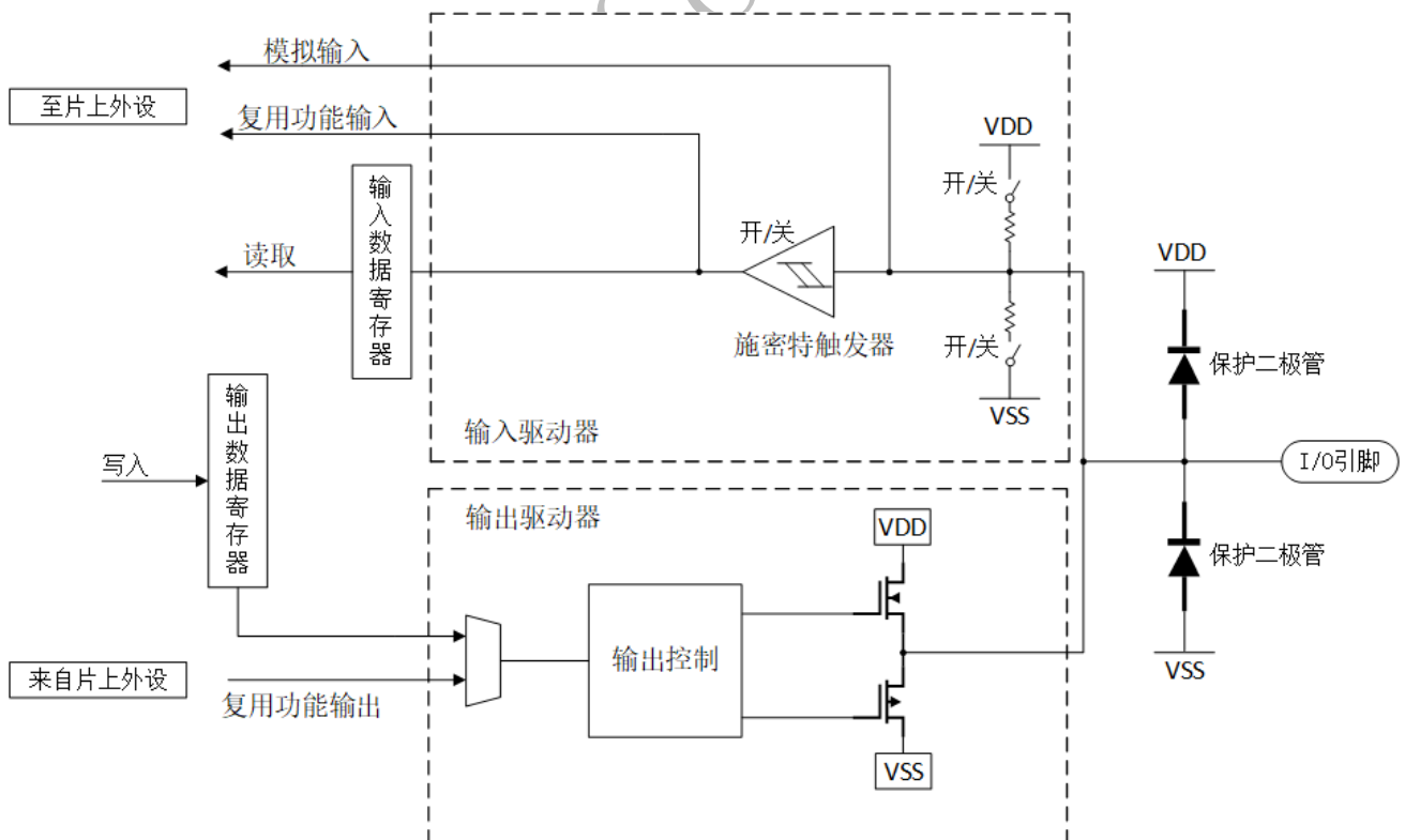
图 3-1 GPIO 结构框图
