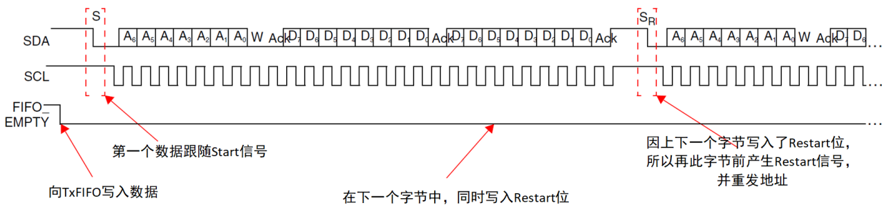
图 8-11 主机发送并产生 Restart 时序
