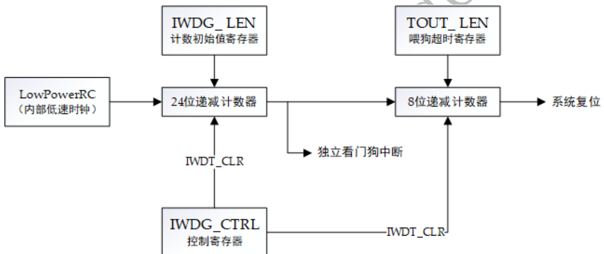
图 14-1 PMU_IWDG 系统框图
