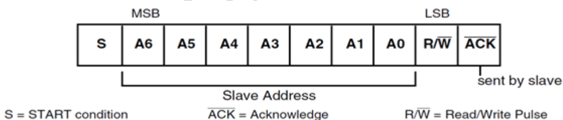
图 8-5 7bit 地址示意图
