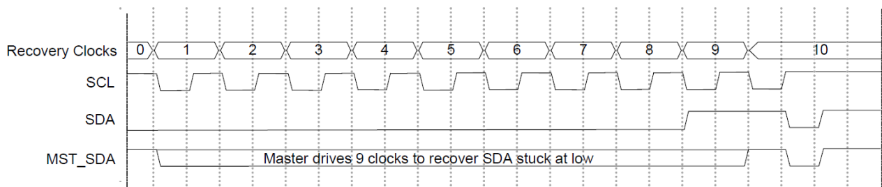
图 8-4 主机发送 9 个 CLK 试图恢复 SDA
