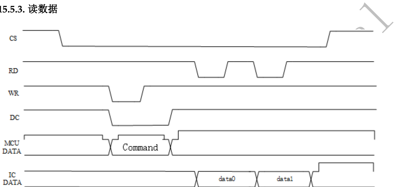
图 15-4 8080 读数据时序
