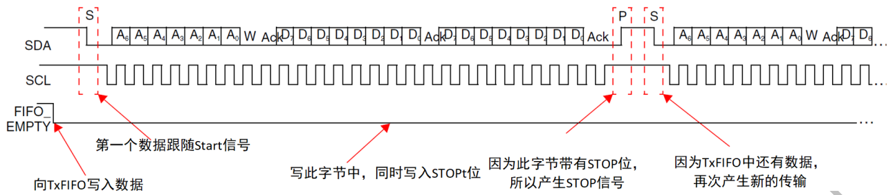
图 8-13 主机发送, 产生 STOP, Tx FIFO 非空
