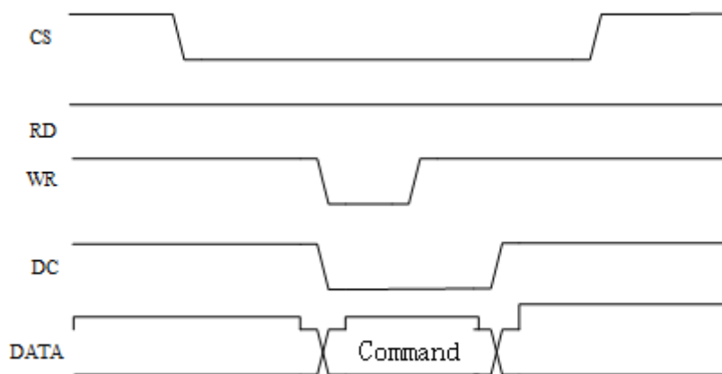
图 15-2 8080 写命令时序
