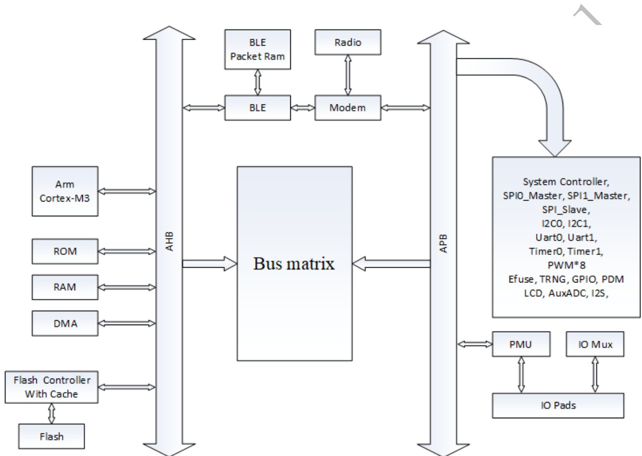
图 1-1 系统框图
