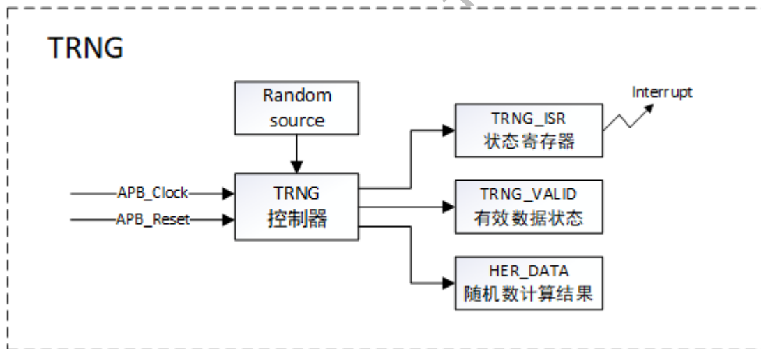
图 10-1 TRNG 结构框图
